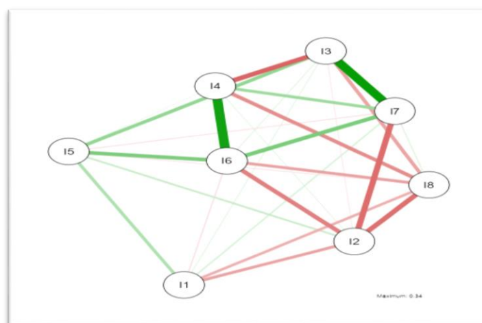
Figura 2. Análisis de redes de correlaciones de los ítems del BISQ
