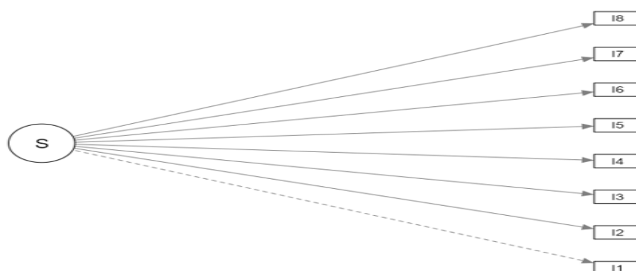
Figura 3. Modelo del BISQ en población ecuatoriana
